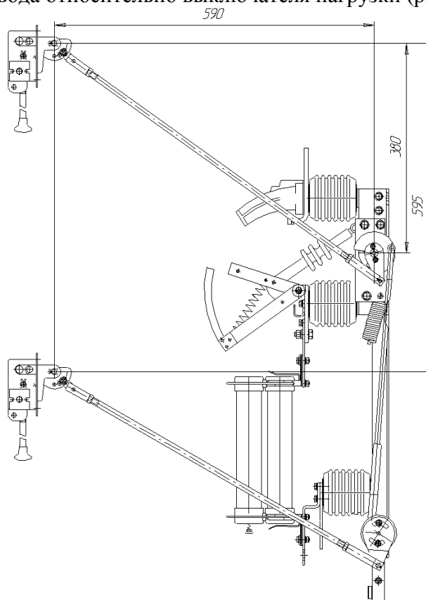
Рисунок 4 – Верхнее расположение приводов относительно валов ВНА
