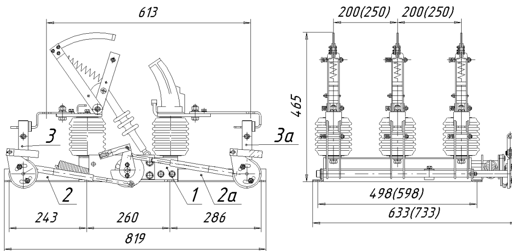
Рисунок 9 - ВНАП-10/630-20-2зУ2.
