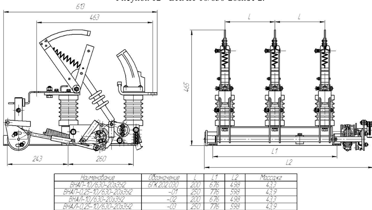
Рисунок 12 - ВНАП-10/630-20з-3пУ2.
