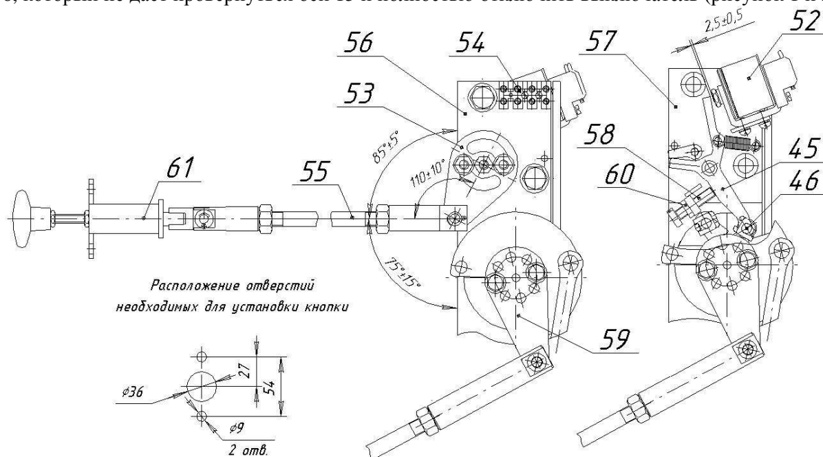
Рисунок 2 – Механизм автоматического и дистанционного отключения ВНА.
