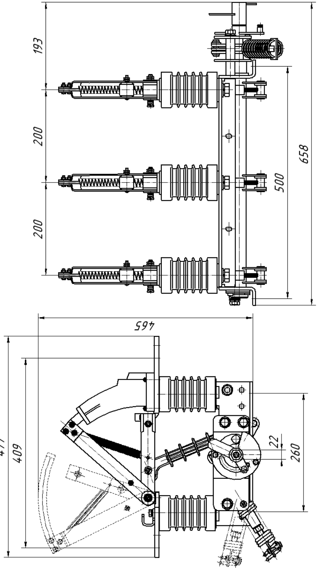
Рис. 16 ВНА СЭЩ Пр-10/630-2042 остальное см. на рис. 1.
