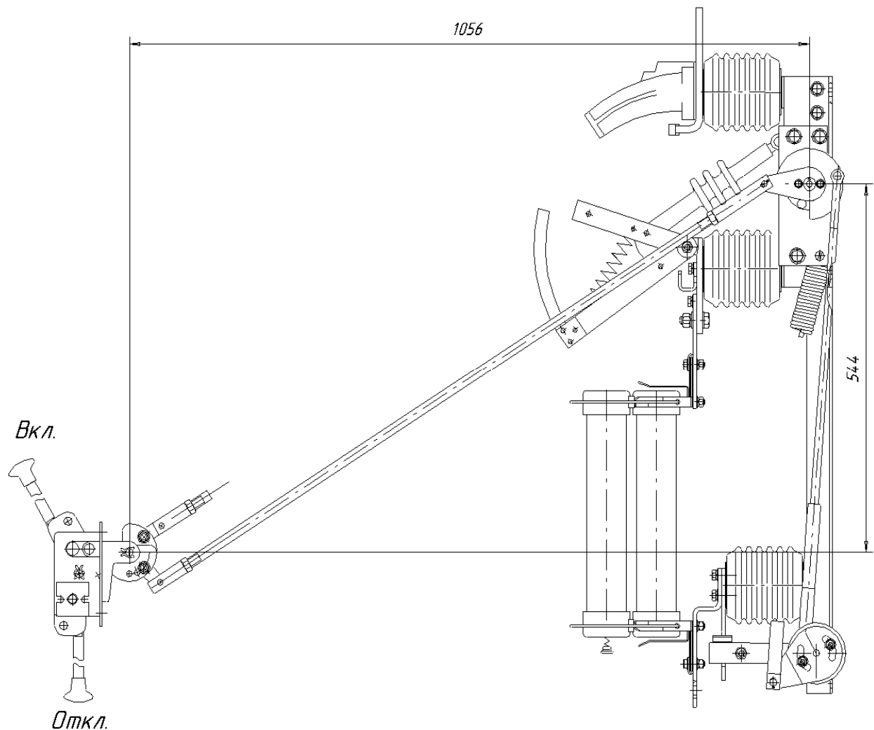
Рисунок 4а – Нижнее расположение привода относительно вала ВНА
