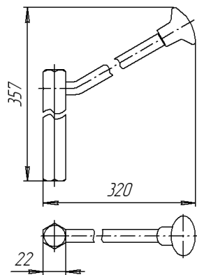
Рисунок 14 – Рычаг шестигранный.
