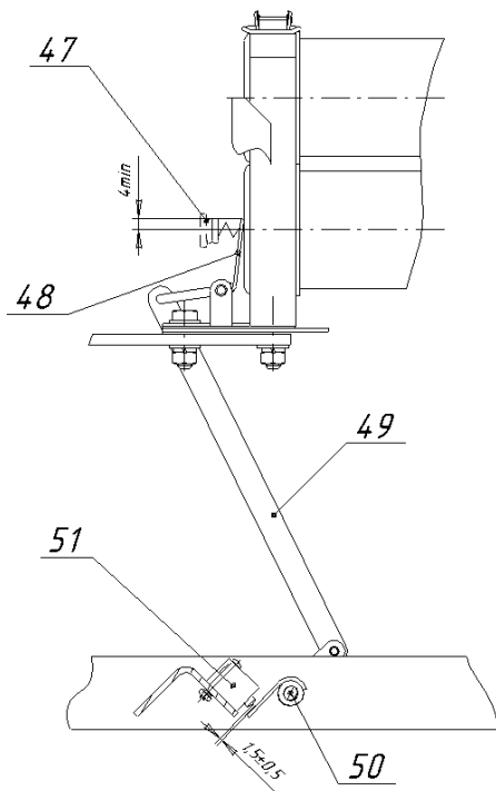
Рисунок 3 – Механизм автоматического отключения при перегорании предохранителей.
