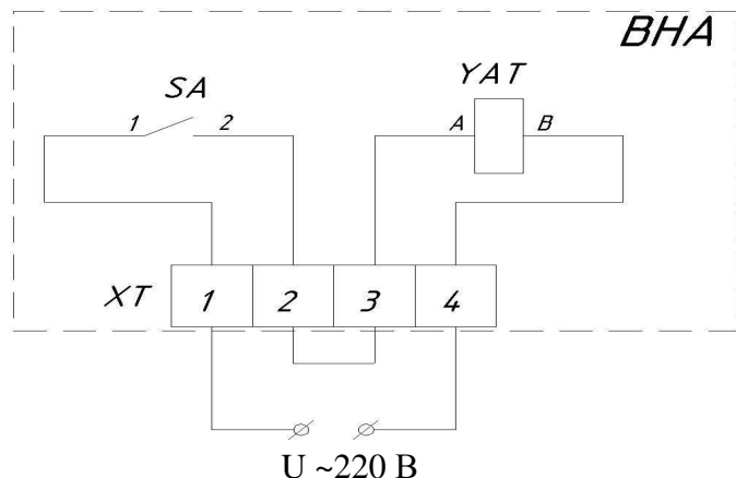
Схема 1: для ВНА-10/630-20-зпЗУ2.
