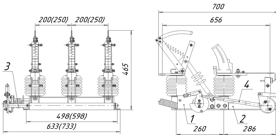
Рисунок 8 - ВНАП-10/630-20-з(св)У2.
