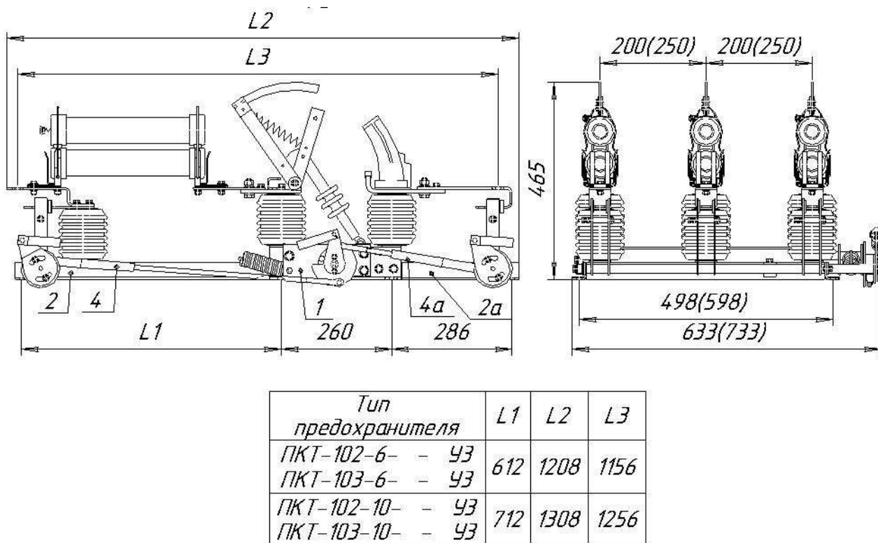
Рисунок 11 - ВНАП-10/630-20з-зпУ2.
