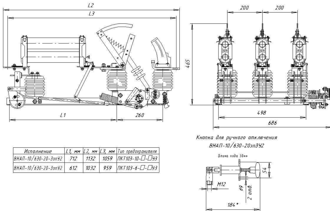
Рисунок 12 - ВНАП-10/630-20з-3пУ2.
