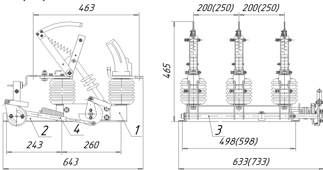
Рисунок 7 - ВНАП-10/630-20зУ2.
