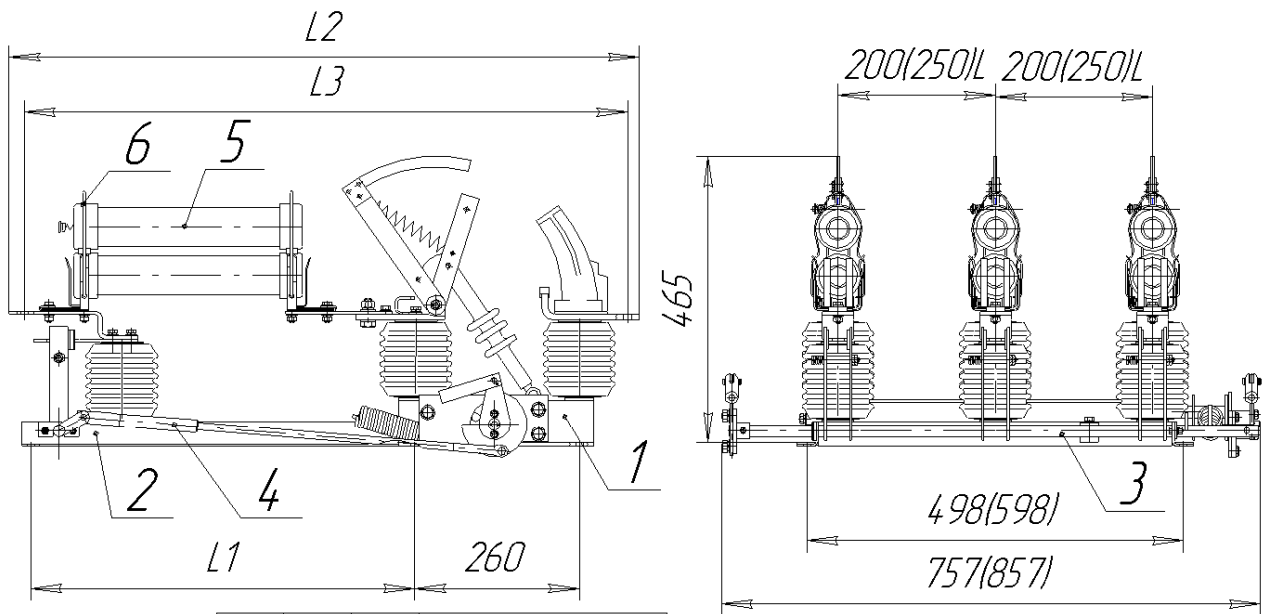
Рисунок 5 - ВНАП(л)-10/630-20зУ2.
