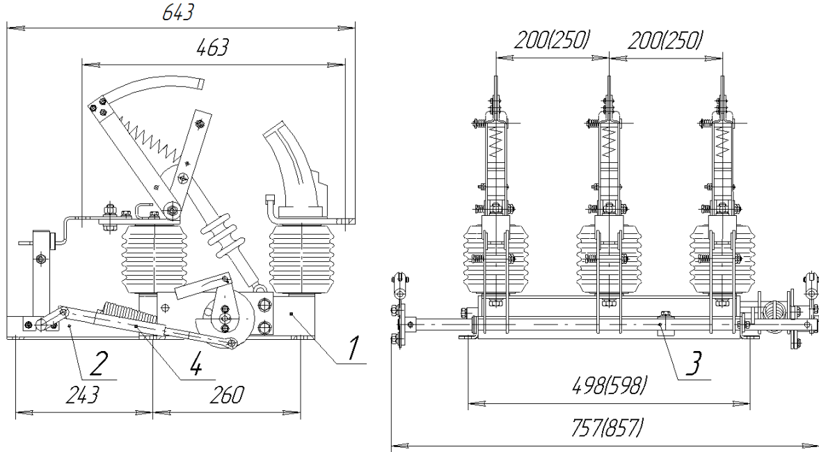
Рисунок 5 - ВНАП(л)-10/630-20зУ2.
