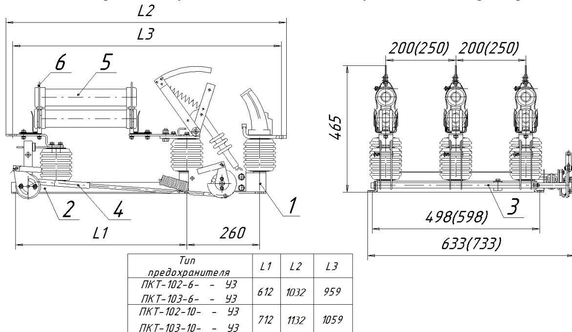
Рисунок 10 - ВНАП-10/630-20зпУ2.
